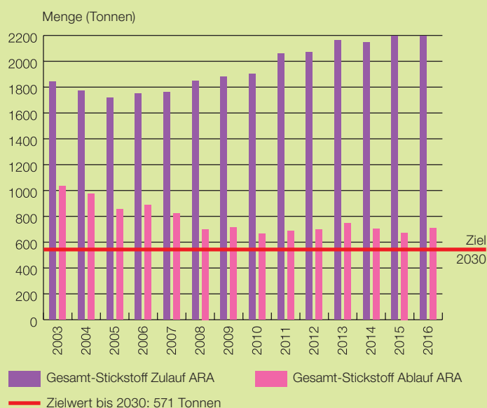
Abb. 21: Zu- und Ablauf von Gesamt-Stickstoff in sämtlichen ARA, Kanton Luzern (2003 bis 2016, Ziel 2030), Quelle: uwe
