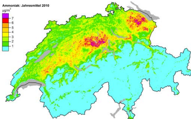
Abb. 9: Luftbelastung durch Ammoniak in der Schweiz (2010), Quelle: bafu
