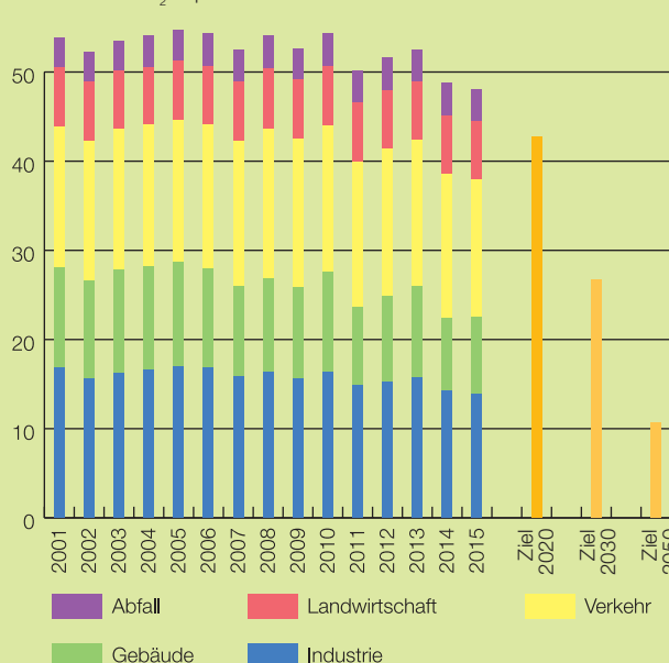
Abb. 26: Treibhausgasemissionen der Schweiz (2001 bis 2015 und Ziele 2020, 2030 und 2050). Quelle: bafu
