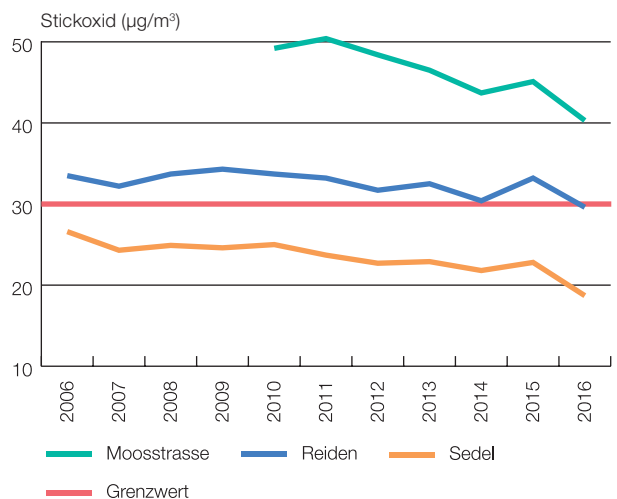
Abb. 22: Durchschnittliche Stickoxidkonzentration an der Moosstrasse in Luzern, in Reiden und auf dem Sedel (2006 bis 2016). Der Grenzwert von 30 \mu\text{g}/\text{m}^3 wird innerstädtisch nicht eingehalten. Quelle: in-luft
